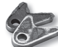
Удаление большого грата (после кислородной резки)
