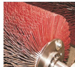
Скругление (2 щетки с абразивной лентой)
