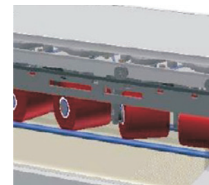
Равномерное скругление всех кромок (Модуль Spin с 3 горизонтально и вертикально вращающимися абразивными щетками с функцией осцилляции)
